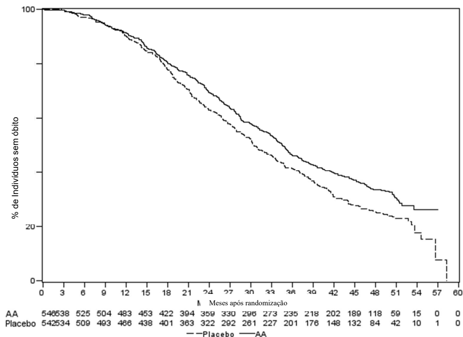
Figura 9: Curvas de sobrevida pelo método de Kaplan-Meier em pacientes tratados com ZYTIGA® ou placebo em combinação com prednisona ou prednisolona associados a agonistas de LHRH ou orquiectomia prévia, análise final
