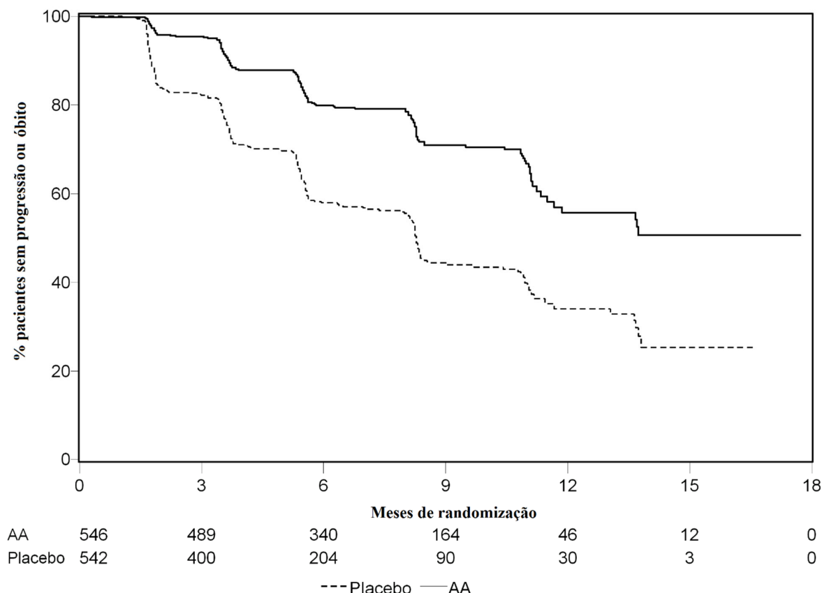
Figura 7: Curvas de sobrevida livre de progressão radiográfica pelo método de Kaplan-Meier em pacientes tratados com ZYTIGA® ou placebo em combinação com prednisona ou prednisolona associado a agonistas de LHRH ou orquiectomia prévia.
