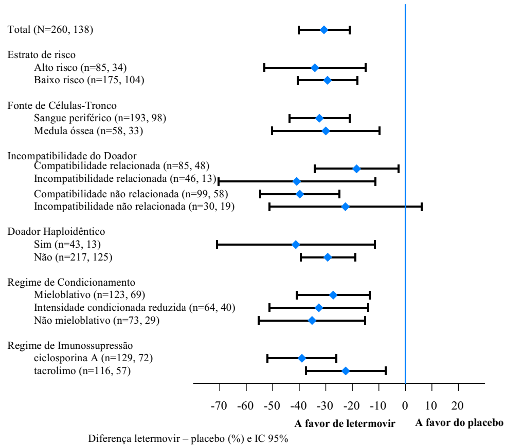
Figura 2: Estudo P001: Gráfico de Forest da Proporção de Indivíduos com Infecção pelo CMV clinicamente significativa até Semana 24 Pós-TCTH por Subgrupos Seleccionados (Abordagem DAO, População FAS)
