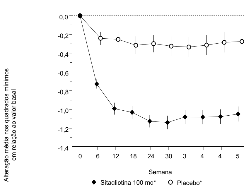
Figura 4: Alteração média da HbA 1c (%) durante 54 semanas em um estudo de sitagliptina como terapia de adição em pacientes não controlados adequadamente com a associação de metformina e rosiglitazona †
